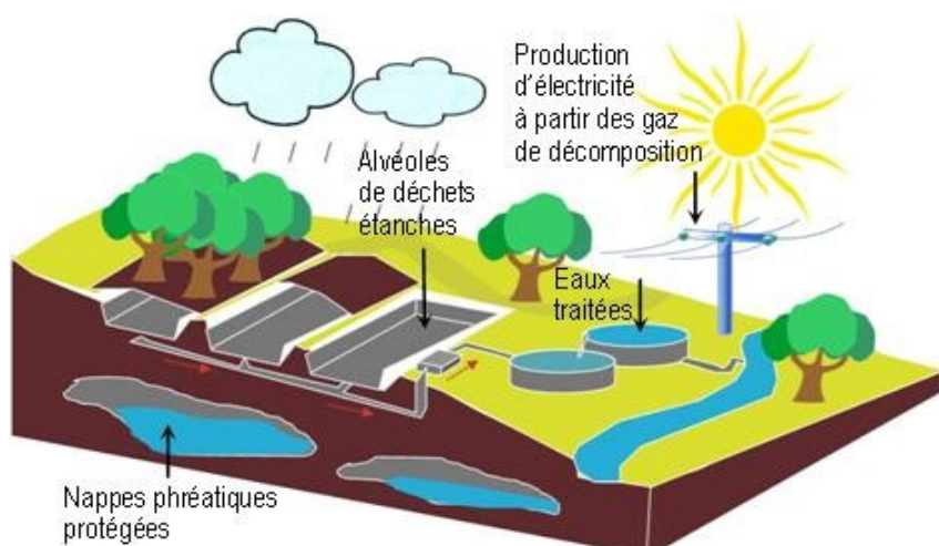
Schéma de principe du centre d'enfouissement
